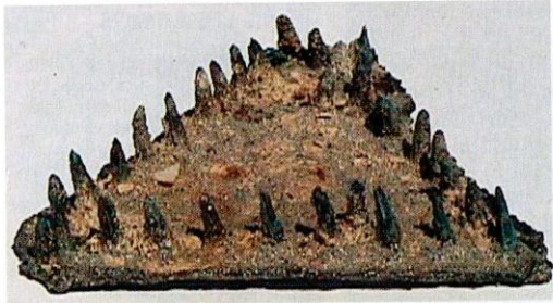
3. CETTE PLAQUE DE CUIVRE CLOUTÉE DE BRONZE (à gauche) est l'un des éléments du revêtement de cuivre du bateau. À la fin du XVIII e siècle, on commence à recouvrir les coques de protection contre les tarets, ces mollusques bivalves à corps allongés en forme de vers, que
